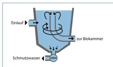
Vortexkammer
