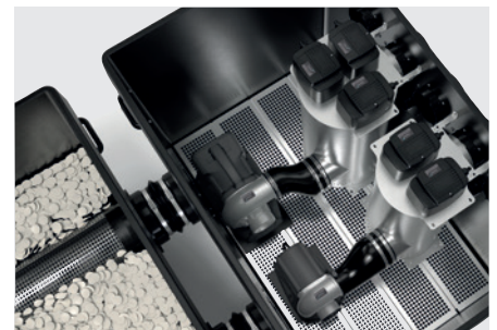
Pumpenkammer: Optimal in das ProfiClear Premium System integrierbar.
