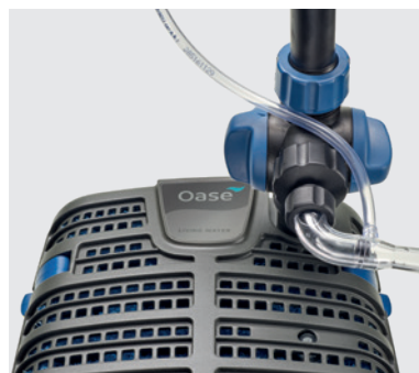
Innovative Belüftungsfunktion: Die Belüftungsdüse sorgt für zusätzlichen Sauerstoffeintrag. Ebenfalls wird eine leichte Strömung im Teich erzeugt, was zu optimalen Filterresultaten führt.
