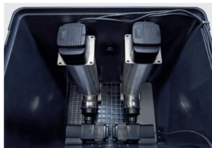
Ablaufmodul Gravitation XL: Vergrößerte Pumpen- und UVC-Kammer zur einfachen Integration von AquaMax Eco Expert und AquaMax Eco Titanium Filterpumpen sowie der neuen Bitron Premium UVC-Vorklärgeräte
