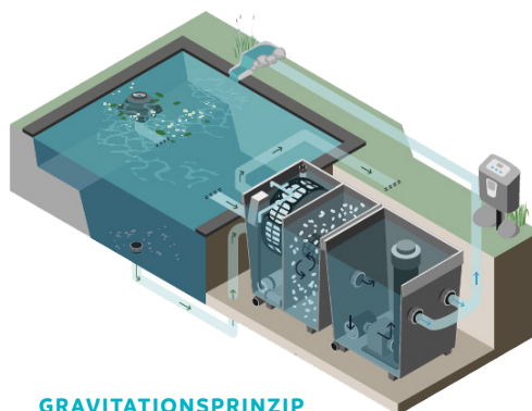
GRAVITATIONSPRINZIP
