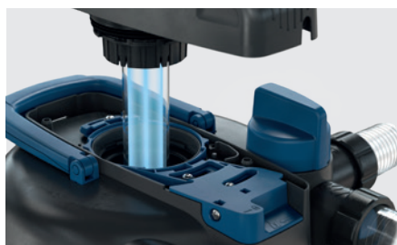
Einfacher Lampenwechsel: Zum Austausch der integrierten UV-Lampe kann das UV-Gehäuse einfach im laufenden Betrieb herausgenommen werden.
