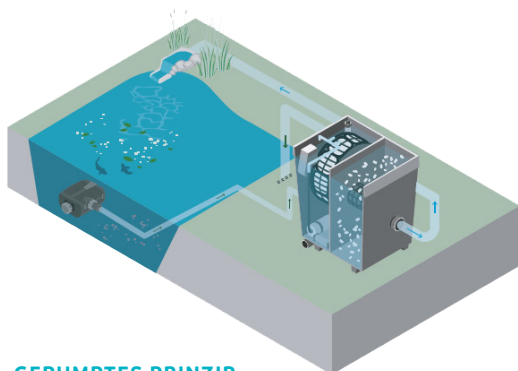
GEPUMPTES PRINZIP
