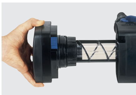
Verschluss-technik: Schnellverschluss zum leichten Öffnen des Lampengehäuses. Ein Sicherheitsschalter deaktiviert die UVC-Lampe hierbei automatisch zum Schutz vor Augenschädigung.
