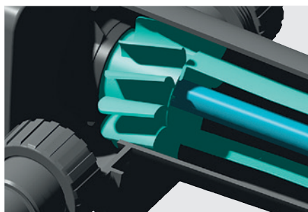
Automatischer Reinigungsrotor: Durch den Wasserstrom wird der Reinigungsrotor kontinuierlich um die Quarzglasröhre herumgeführt und verhindert so Schmutzablagerungen.
